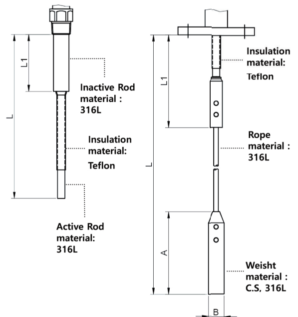
Rod Probe
