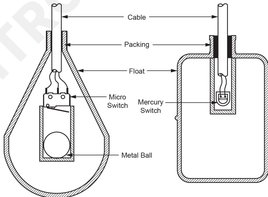
[ Micro S/W Float의 내부 구조도 ]
