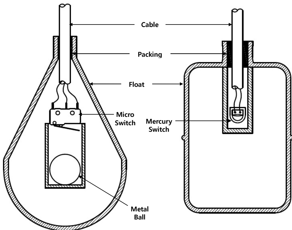
&lt;Micro S/W Float의 내부 구조도&gt;
