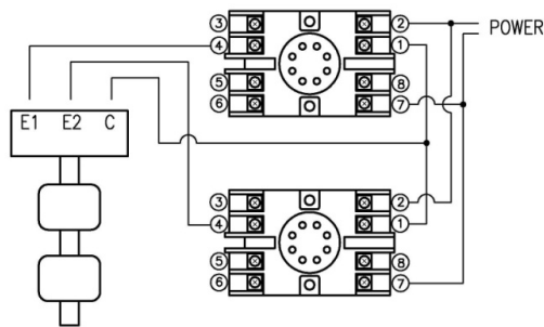
HLC-200Ax2 2-SPST 접점 결선
